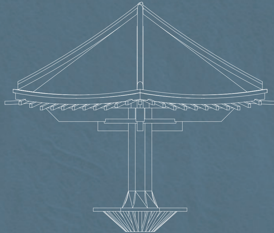
E-1 立面图 1/70
