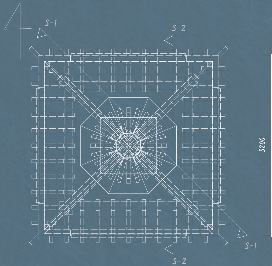
平面图 1/70
