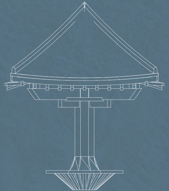
E-2 立面图 1/70
