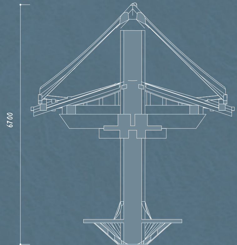
S-2 断面图 1/70
