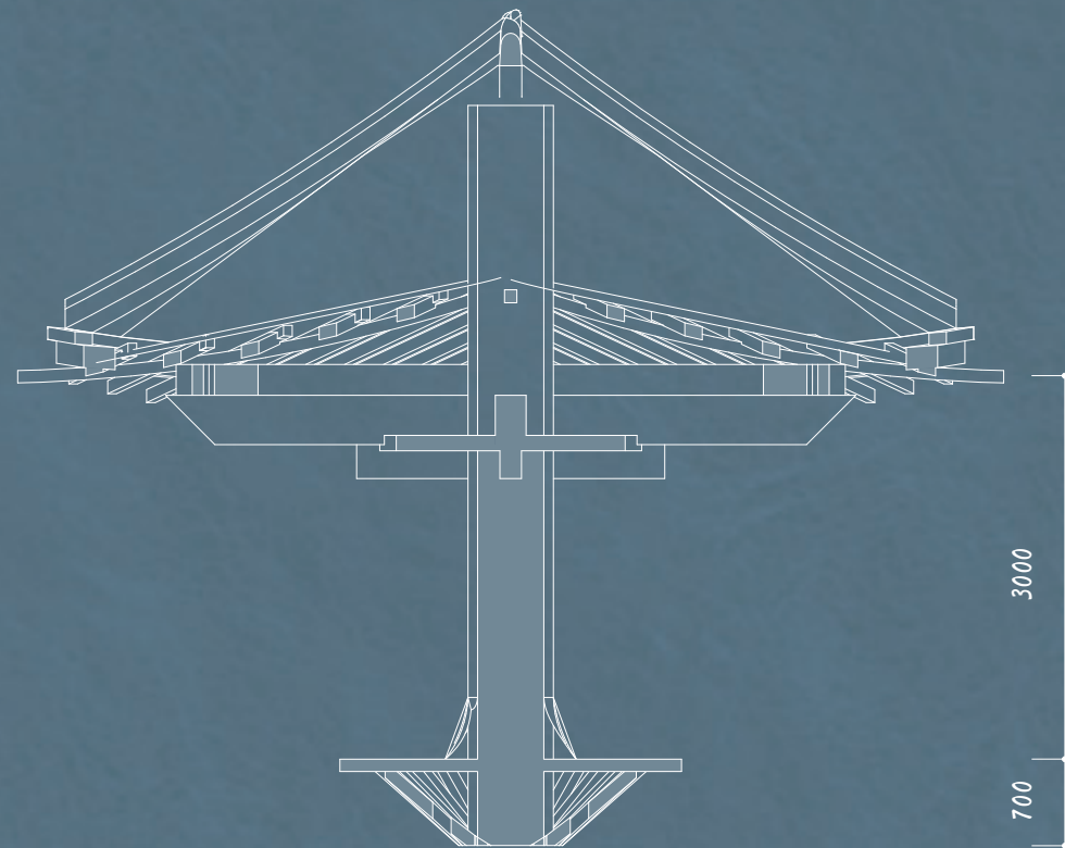
S-1 断面图 1/70
